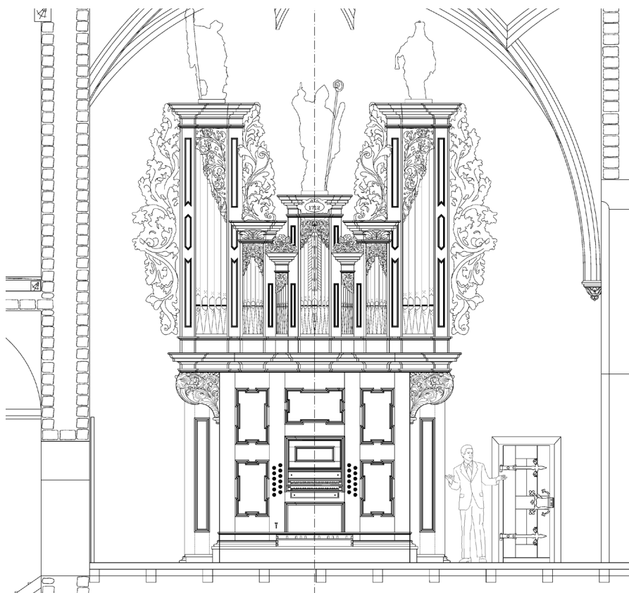
Návrh varhanní skříňe pro kostel sv. Petra a Pavla (za využití barokního prospektu), Varhanářská dílna Kánský – Brachtl, sdružení, 2012.
