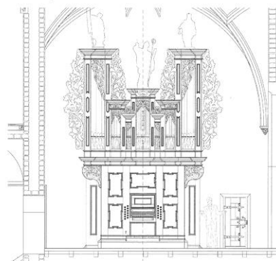
Návrh varhanní skříňky pro kostel sv. Petra a Pavla (za využití barokního prospektu). Varhanní skříň dlna Kánský - Brachtl, sčrtnutí, 2012.
